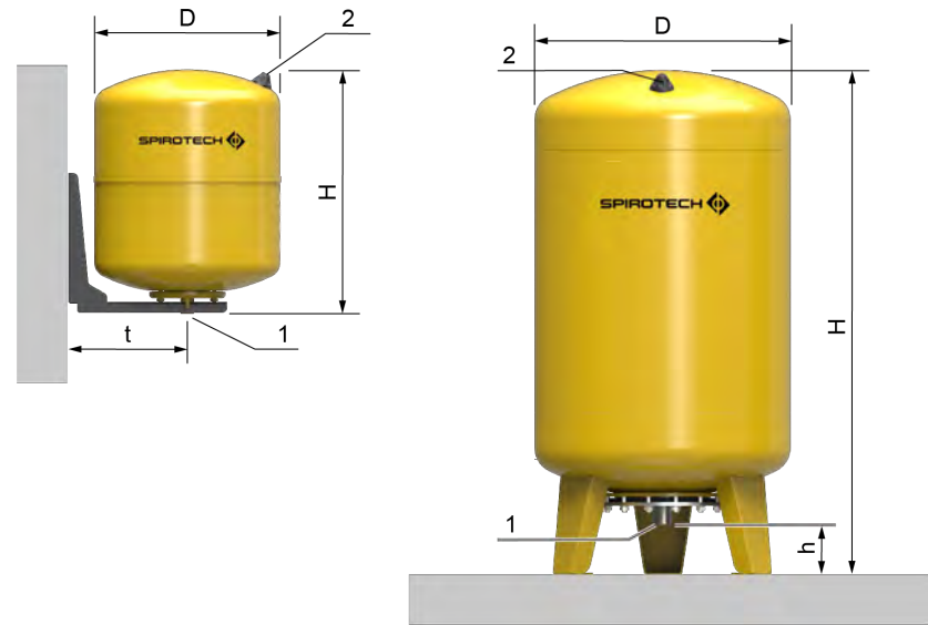
EVU6-18 .. EVU6-50
